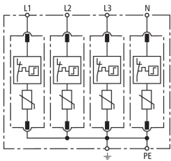
DG M TNS 275 CN 基本线路图
