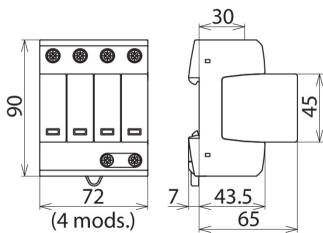
DG M TNS 275 CN 尺寸图
