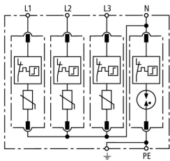
DG M TT 385 CN 基本线路图
