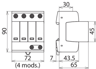
DG M TT 385 CN 尺寸图
