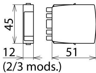
BSP M4 BD 24 尺寸图
