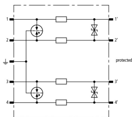
BSP M4 BD 24 基本线路图
